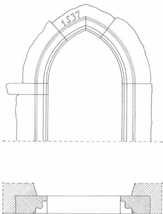
↑ Izris dokumentiranega poznogotskega portala na glavni fasadi grajskega jedra. Pogled in tloris. Poskus rekonstrukcije na osnovi fotografije Cirila Velepčiča iz leta 1947 in skice Ivana Komelja iz leta 1949 (risal: Igor Sapač, 2003).
