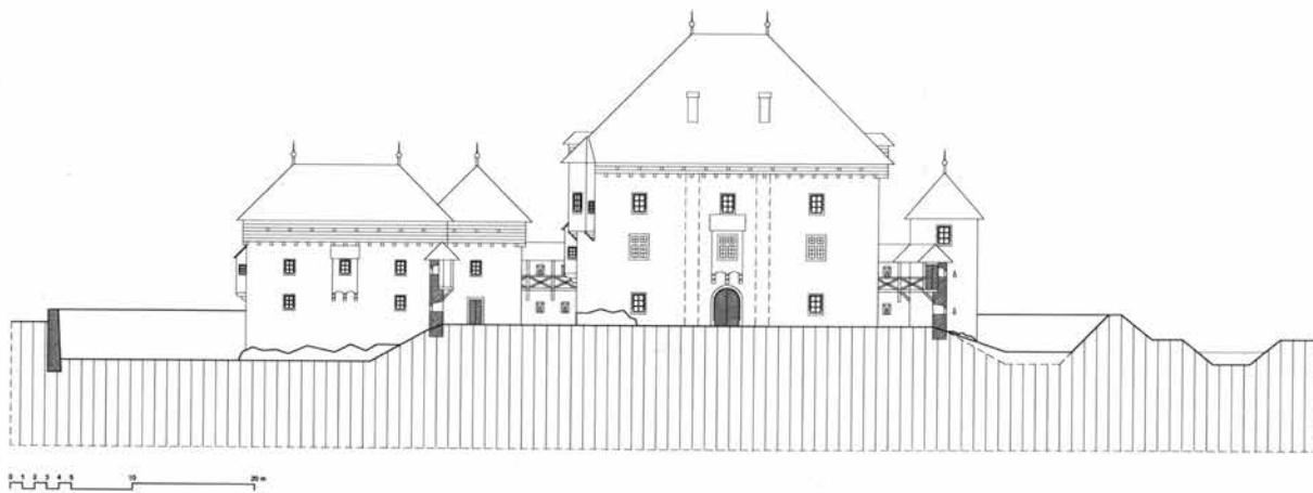
↑ Prerez gradu Breg proti jugovzhodu z glavno fasado glavnega grajskega poslopja. Poskus rekonstrukcije (Igor Sapač. 2018)
