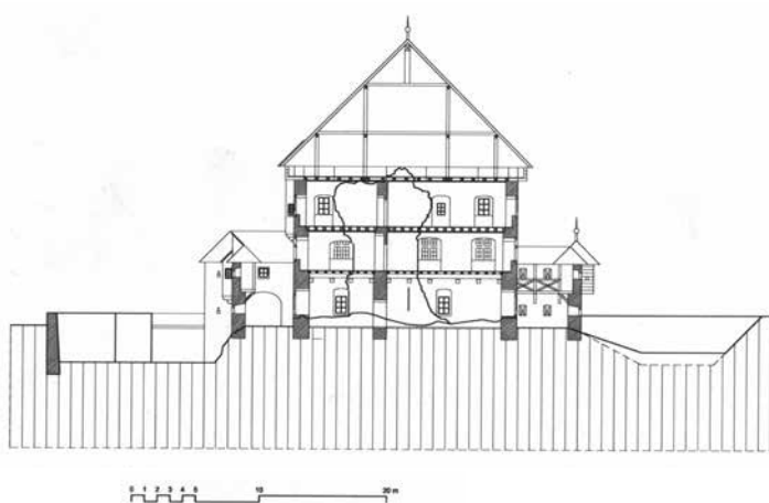
↑ Prerez gradu Breg proti severovzhodu skozi glavno grajsko poslopje. Poskus rekonstrukcije (Igor Sapač. 2018)
