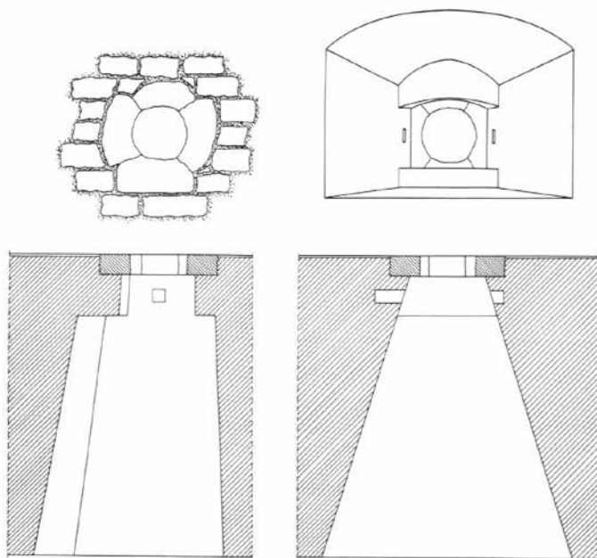
↑ Izris strelne line v pritličju renesančnega južnega stolpa gradu Ortnek. Pogleda od zunaj in znotraj, prerez in tloris. (Igor Sapač, 2003).
