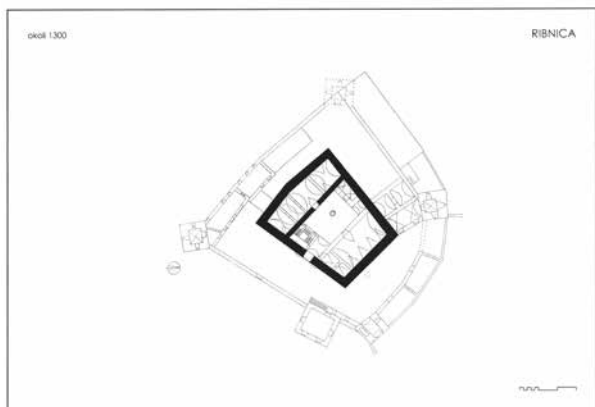
↑ Grad Ribnica okoli leta 1300. Poskus rekonstrukcije. Aksonometrična študija (risal: Igor Sapač, 2003).
