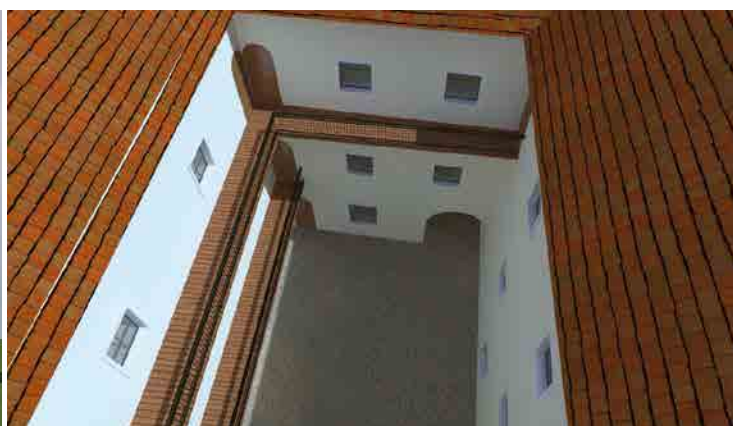
Grad Ribnica okoli leta 1830. Pogled iz zraka proti severozahodni strani dvorišča grajskega jedra. Računalniška študija. Poskus rekonstrukcije (Izdelal Rok Šinko na podlagi risb Igorja Sapača, 2017).
