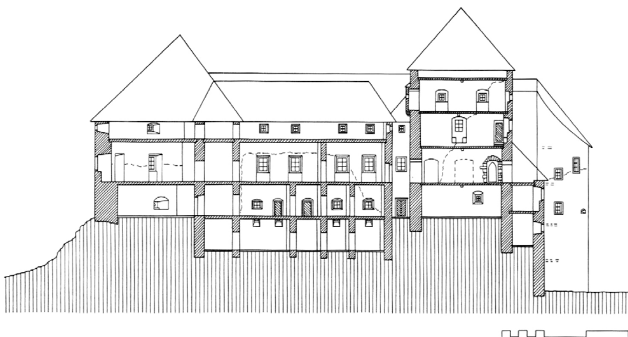
↑ Poskus rekonstrukcije prereza gradu Ortnek pred letom 1884 proti zahodu (Igor Sapač, 1998 in 2003).
