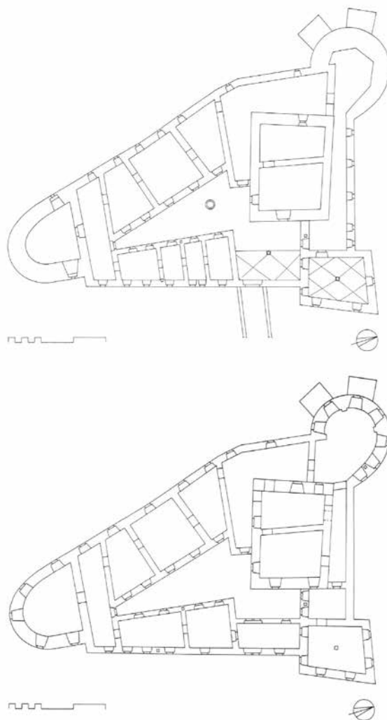
↑ Poskus rekonstrukcije tlorisa pritličja (zgoraj) in prvega nadstropja (spodaj) gradu Ortnek pred letom 1884. Po starejšem načrtu iz arhiva ZVKDS OE Ljubljana dopolnil in izrisal Igor Sapač, 1998 in 2003.
